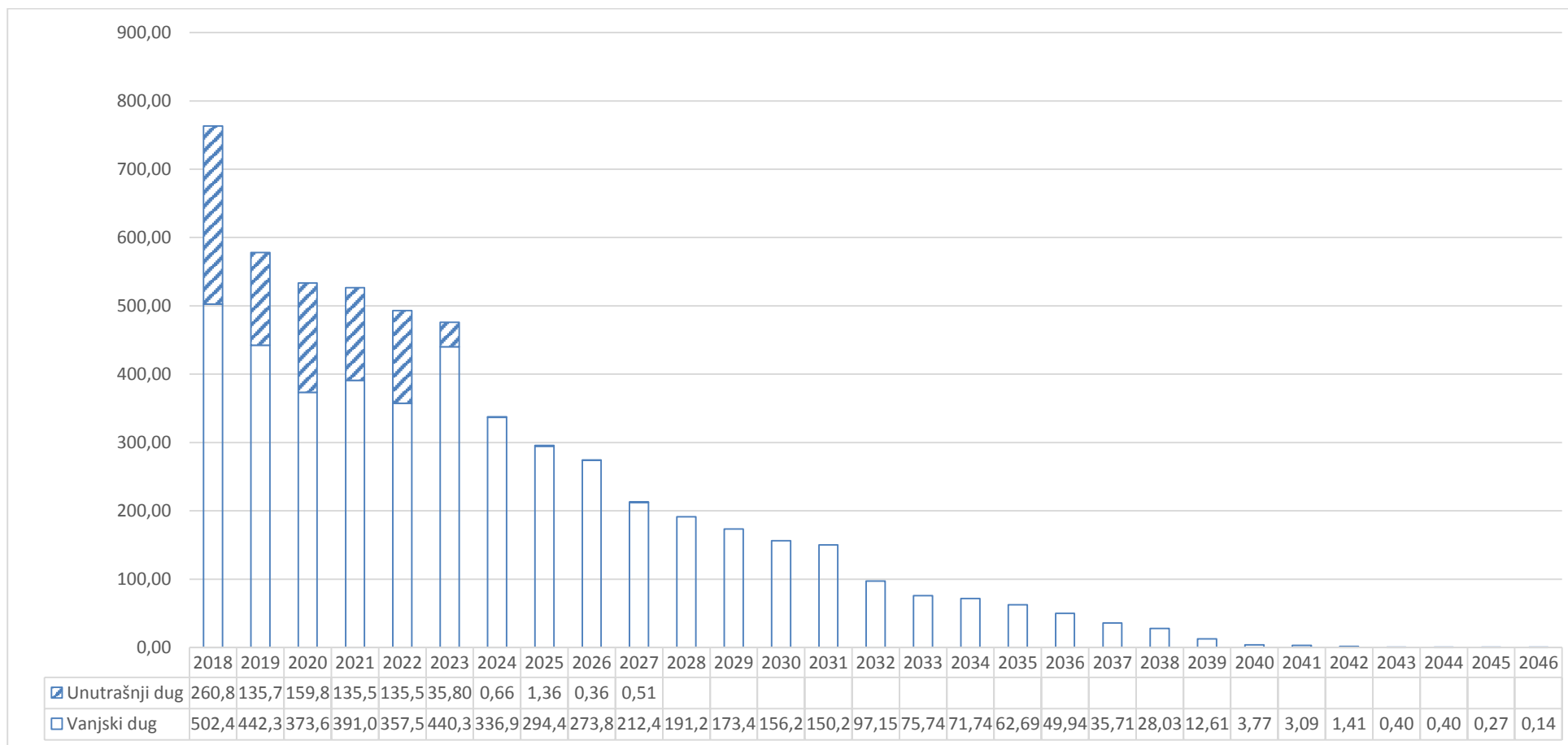
Slika 7. Otplatni profil portfolija duga 12 na dan 31.12.2017. godine
